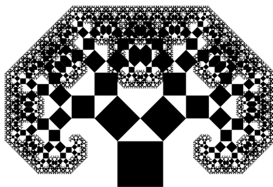
FIGURA 2: Modelo de Fractal Pitagórico Fonte: Wikimedia Commons 9
